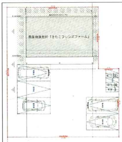
配置計画図
