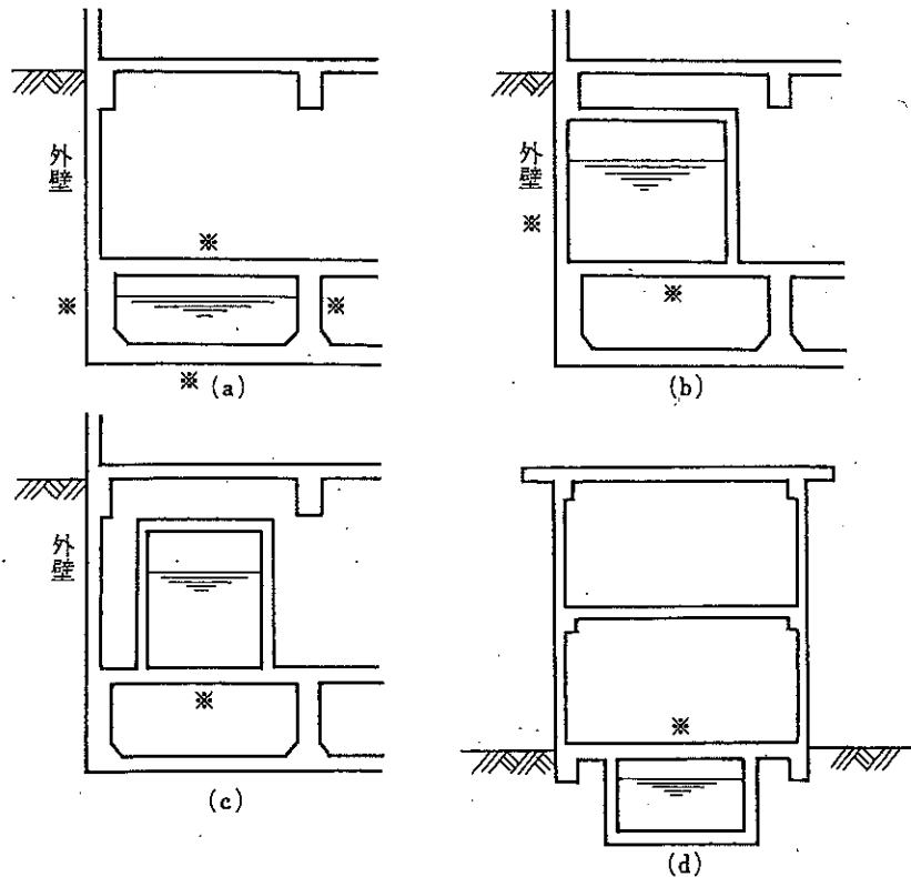
(a), (b), (c), (d)いずれも※の部分が建築物の床スラブや、外壁などを兼用しているの で、第1第二号イの(2)に適合しない。
