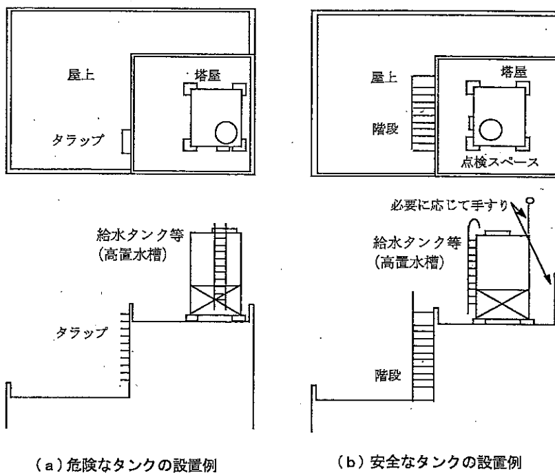
図2-7 給水タンク等（高置水槽）の設置例
