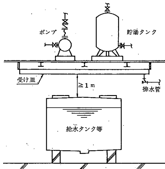
図2-16 給水タンク等の上部に機器類を設置した場合の措置例
