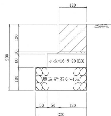
境界断面図 F2-D1
