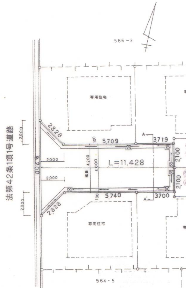
道路平面図
