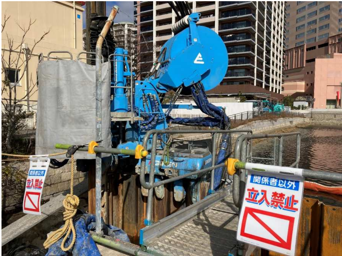
⑥到達立坑を造る準備に着手
