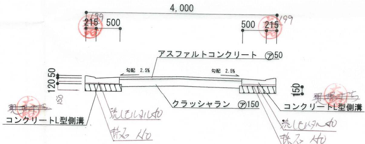
標準横断面図 (S=1 : 50)
