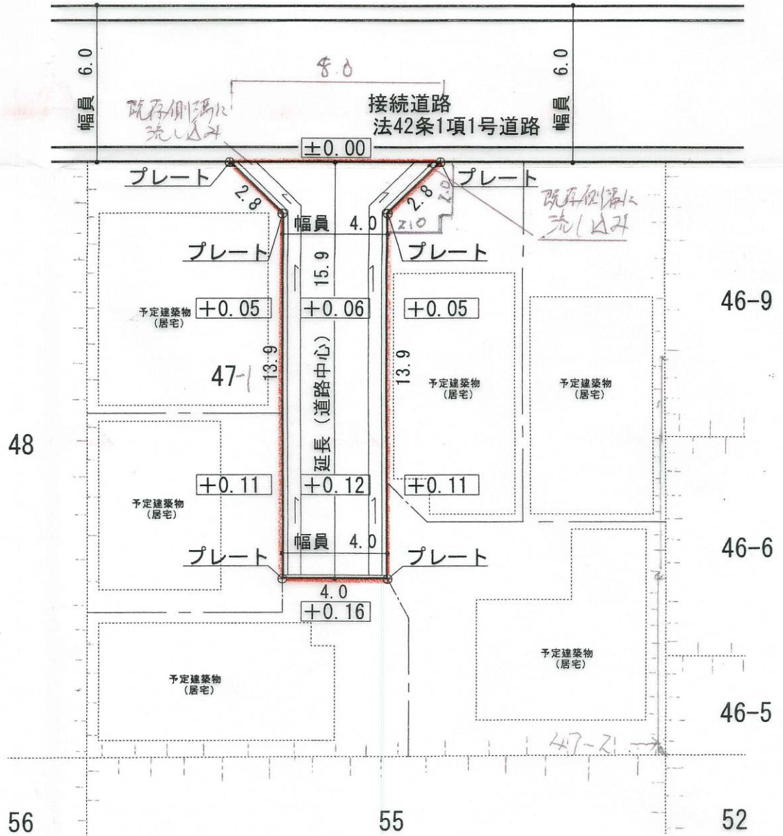
道路図 (平面図) (S=1 : 200)
