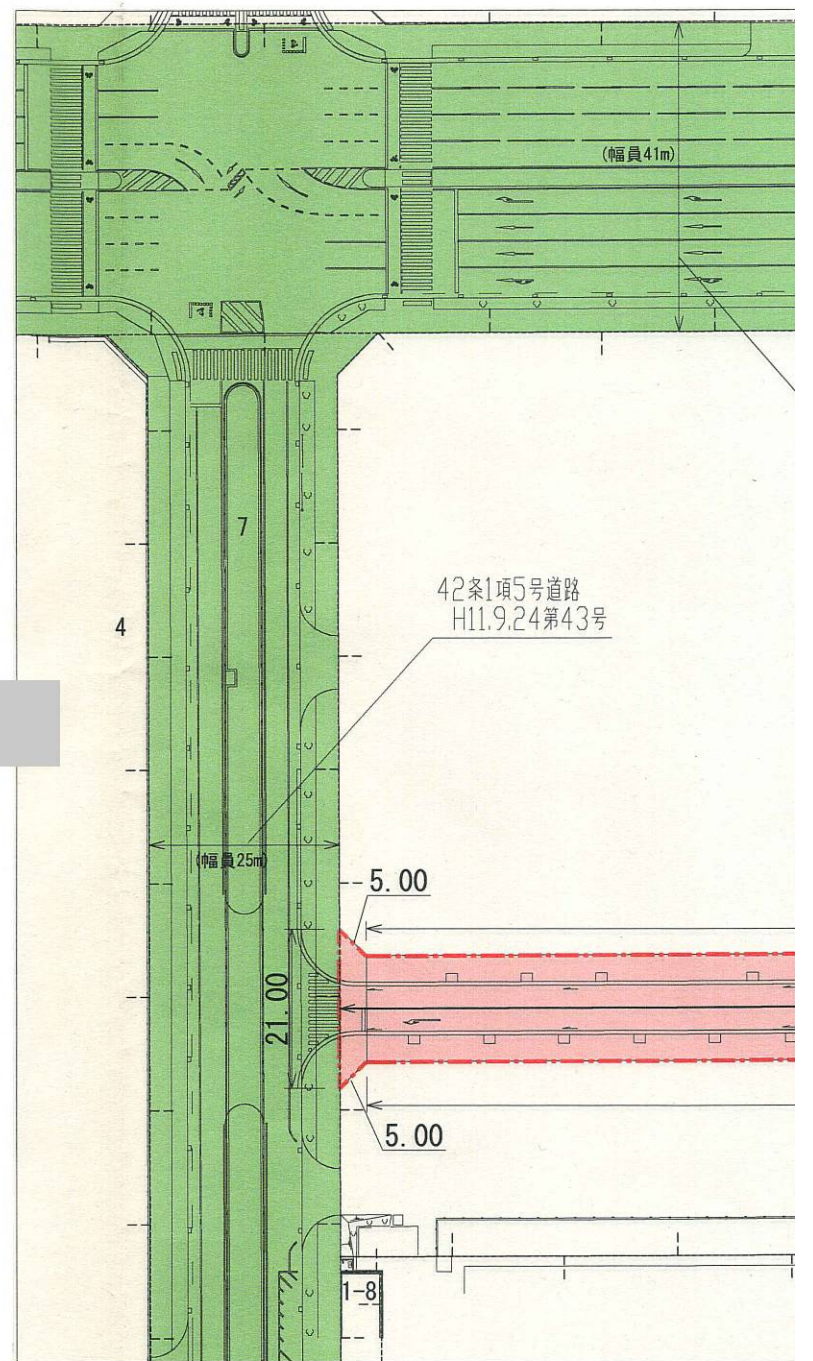
平面図 1/1,000
